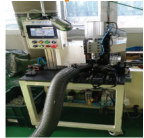
휠 후가공
